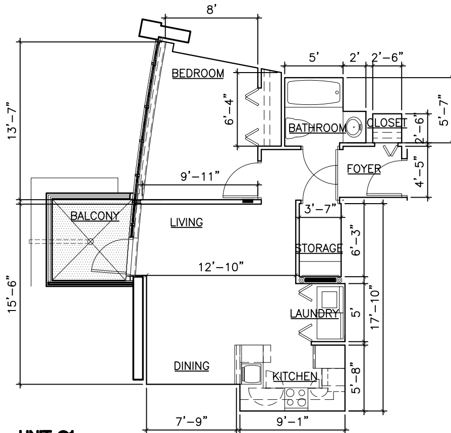
UNIT G1 SCALE: 1:100
