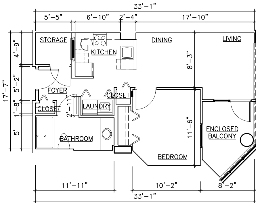
UNIT C1 SCALE: 1:100
