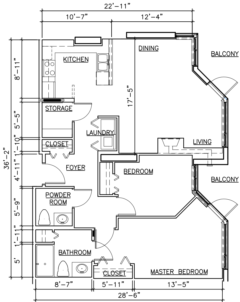
UNIT H1 SCALE: 1:100
