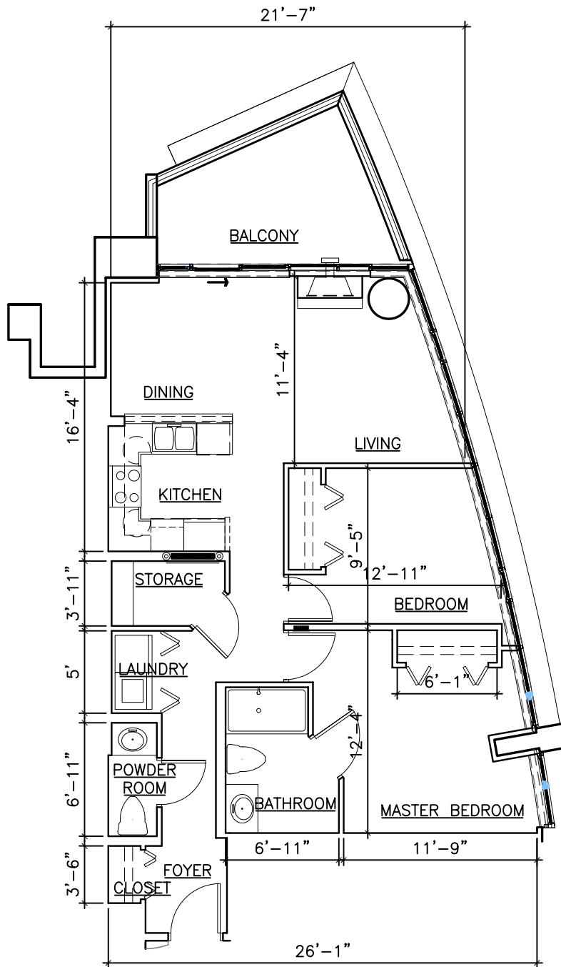
UNIT J1 SCALE: 1:100
